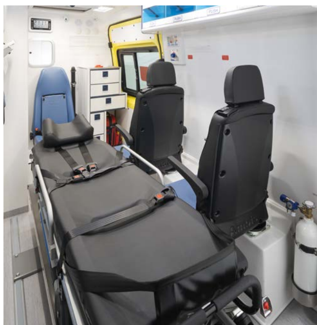
Zwei klappbare Begleitersitze auf der rechten Seite für das Rettungspersonal oder Begleitpersonen.
